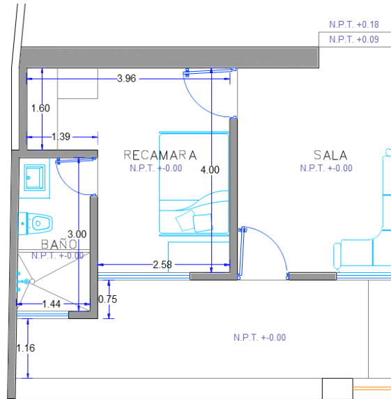
PROPUESTA ESC. 1:50
