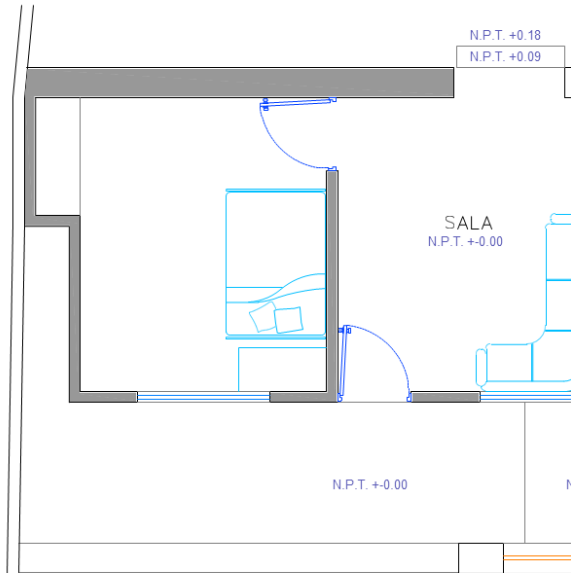
LEVANTAMIENTO ESC. 1:50
